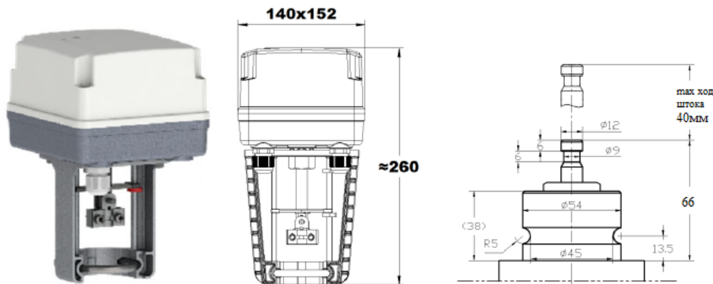
Рисунок 1 – Габаритные размеры Э/П ENCO-310MB-2000/80-40-220B-IP54
