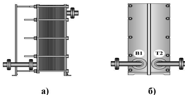
Рис.10 Подключение трубопроводов к нажимной плите теплообменника.
