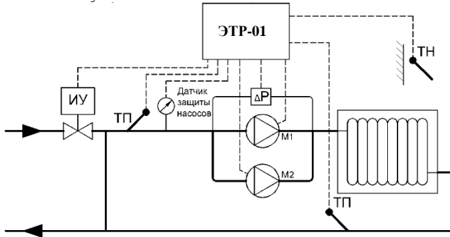
Рисунок Б.1 – Монтажная схема регулятора ЭТР-01 (программа 10) в системе управления зависимым контуром отопления
