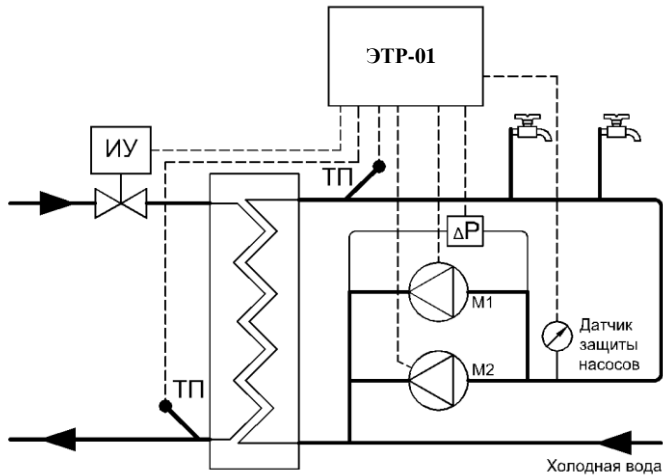
Рисунок Б.3 – Монтажная схема регулятора ЭТР-01 (программа 20) в системе управления контуром ГВС
