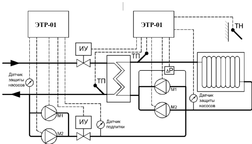
Рисунок Б.2 – Монтажная схема регуляторов ЭТР-01 в системе управления независимым контуром отопления (программа 10) и контуром подпитки (программа 40)
