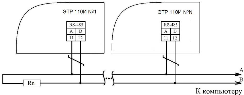
Рисунок 4.1 - Схема подключения ПК к блоку ЭТР с интерфейсом RS-485
